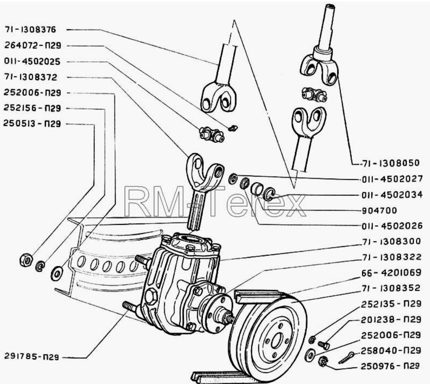
Рис. 37. Вентилятор
