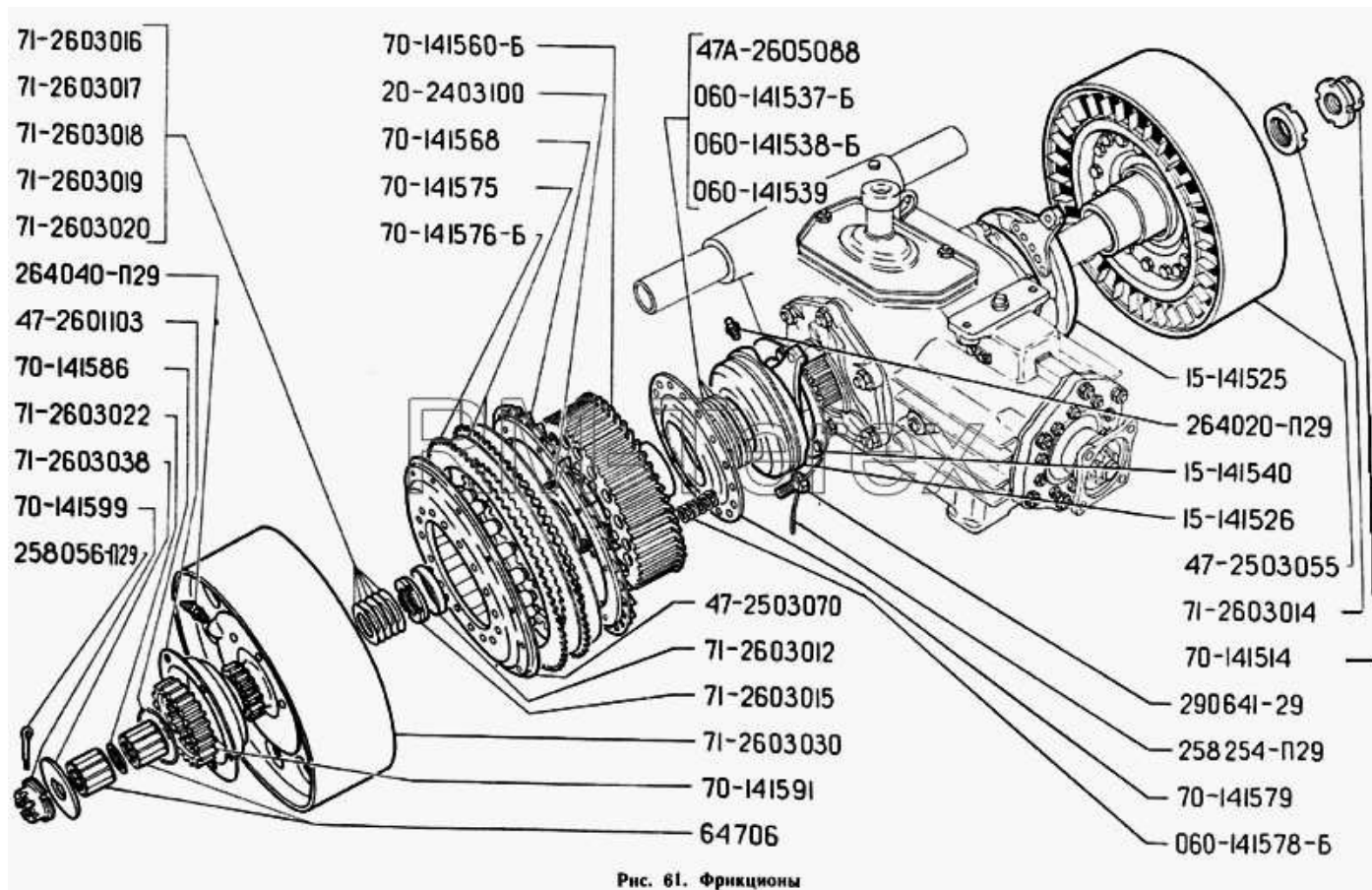
Рис. 61. Фрикционы
