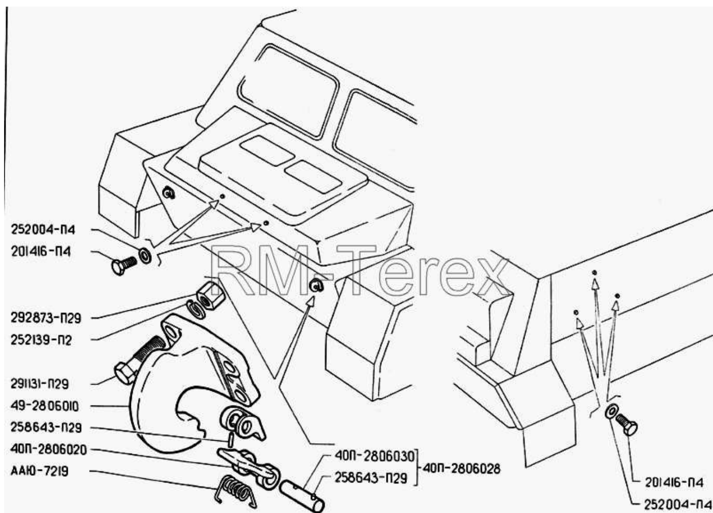
Рис. 67. Передние буксирные крюки и крепление номерных знаков
