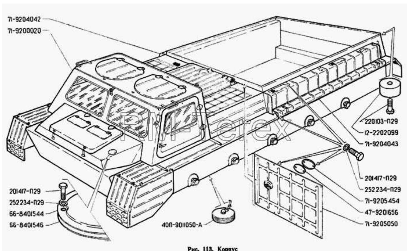
Рис. 113. Корпус
