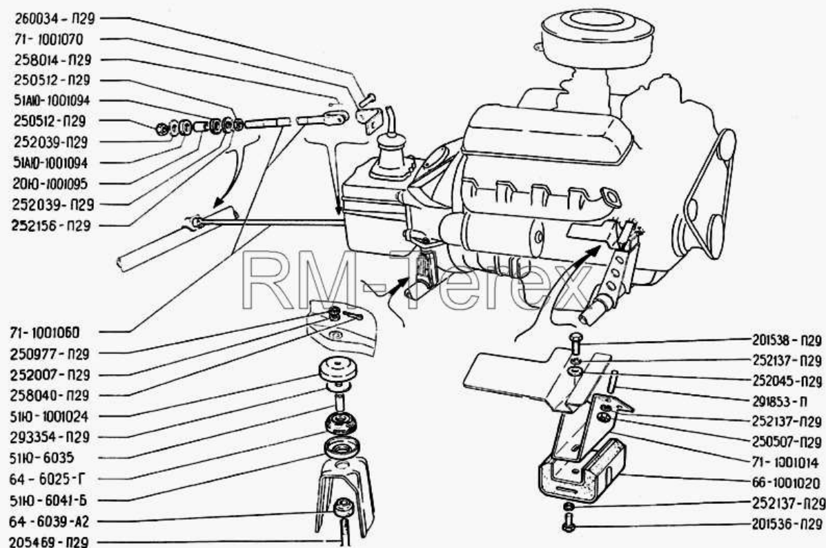
Рис. 2. Подвеска двигателя
