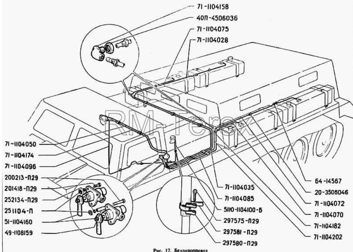
Рис. 17. Бензинопровод.
