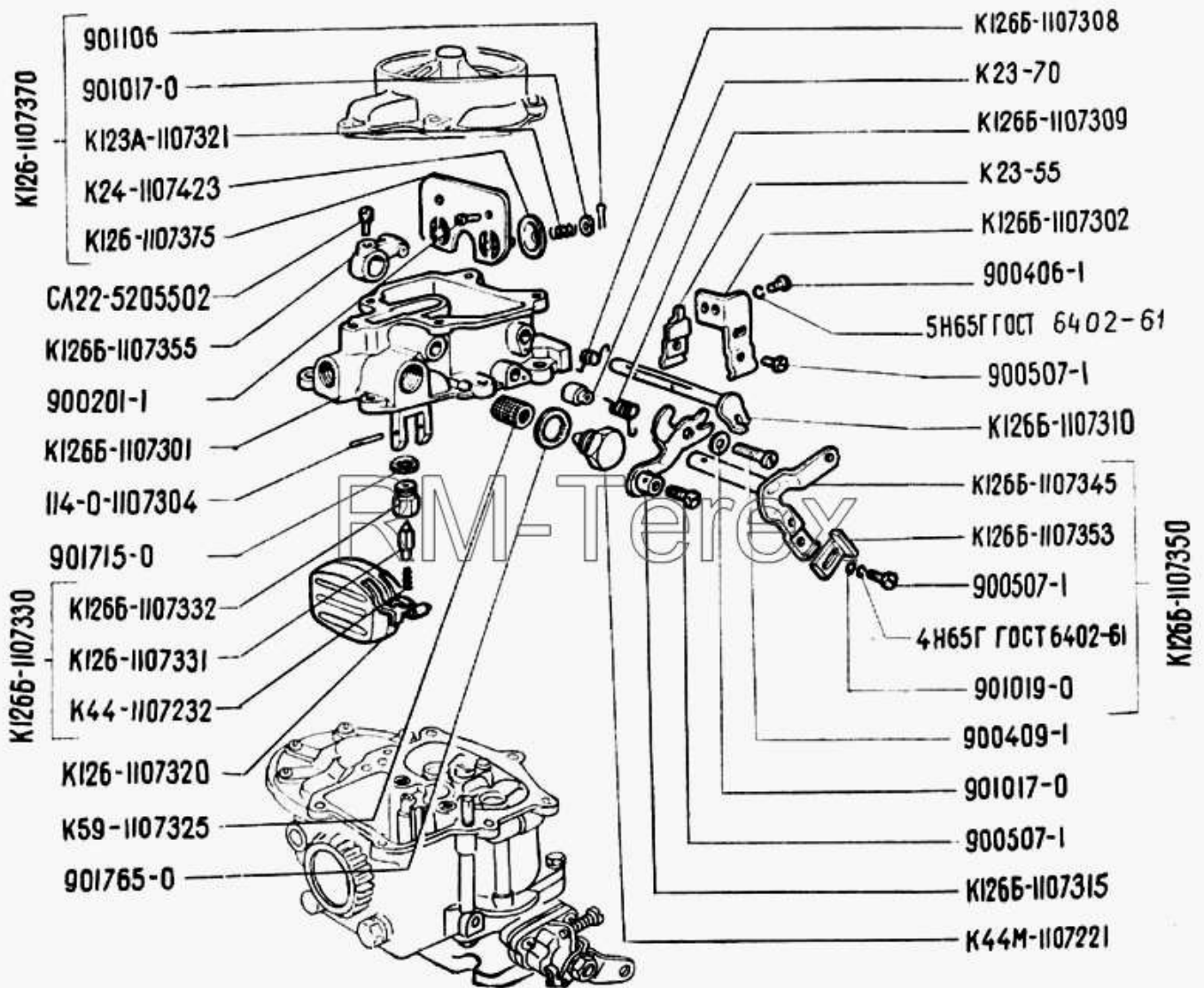
Рис. 23. Карбюратор
