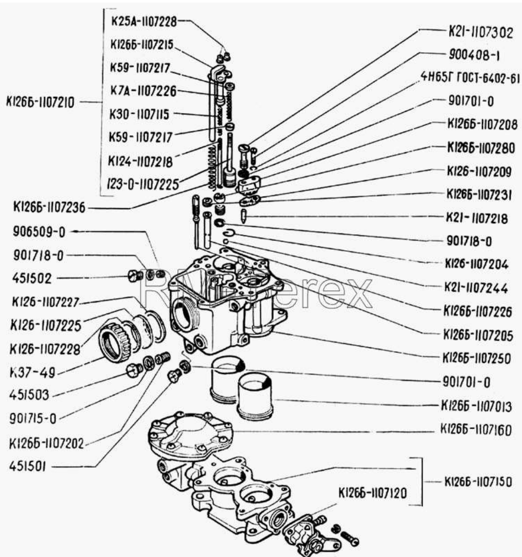
Рис. 21. Карбюратор
