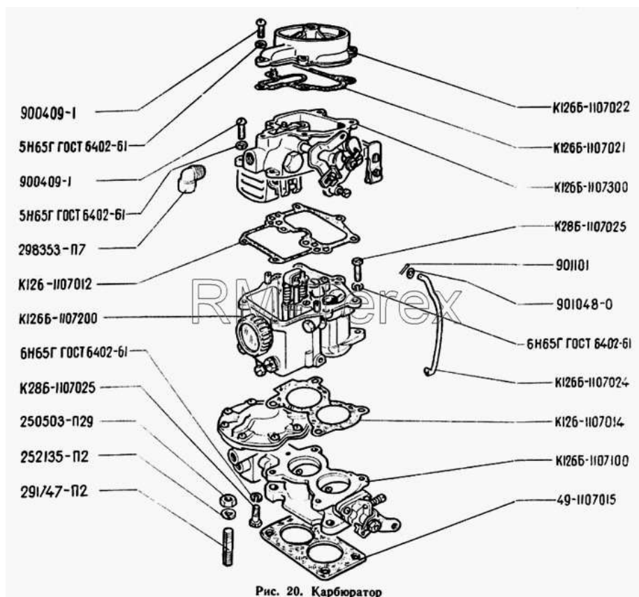
Рис. 20. Карбюратор
